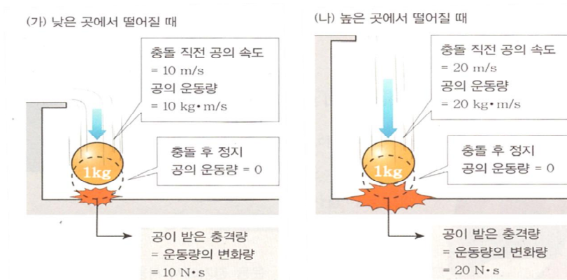
[그림 2] 떨어져 정지하는 공의 충격량
