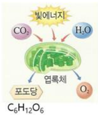
[그림 2] 광합성
