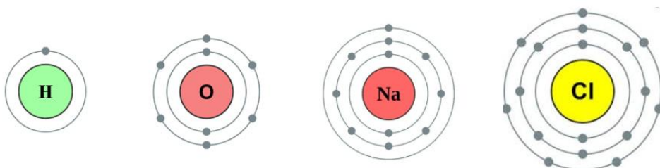
[그림 1] 수소, 산소, 나트륨, 염소 원자 구조
