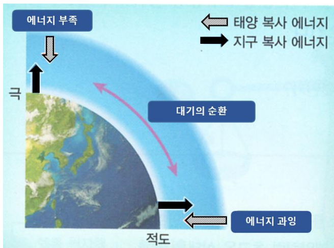
[그림 4] 대기의 순환
