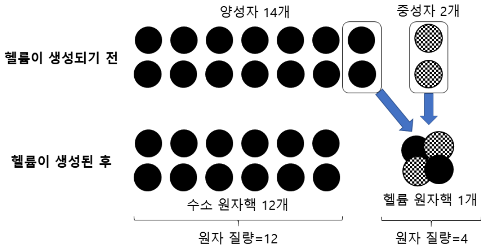
[그림 3] 수소 원자핵과 헬륨 원자핵의 생성 과정
