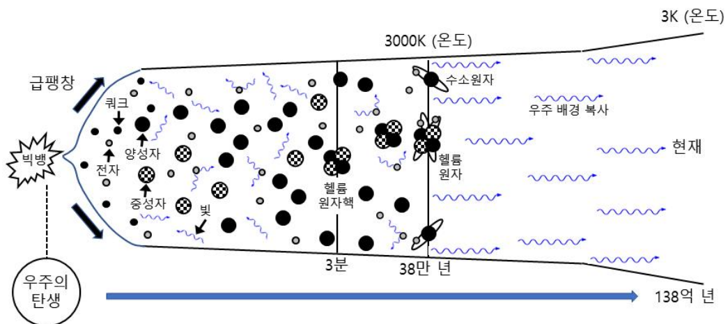
[그림 1] 빅뱅 이후 우주가 팽창하는 과정
