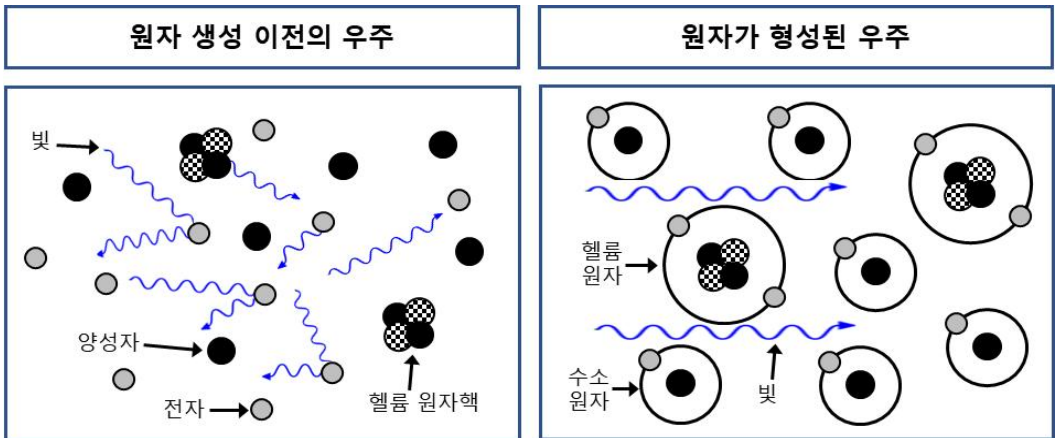
[그림 2] 우주를 구성하는 입자와 빛의 투과성
