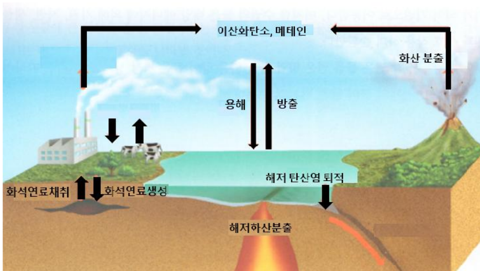
[그림 1] 탄소의 순환
