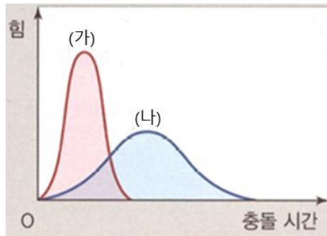
[그림 1] 힘과 충돌 시간의 관계*
